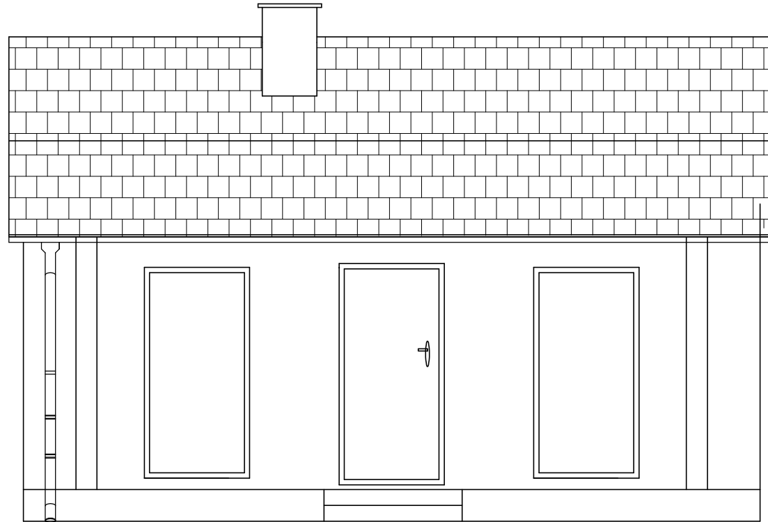
Elewacja północna
